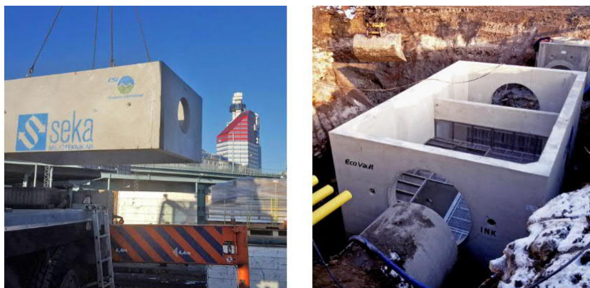
Figur 3. Sedimentationsmagasin med filter. Bildkälla: Seka Miljöteknik.
