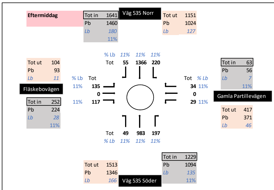
Figur 8 - Dimensionerande trafikflöden i korsningen väg 535-Fläskebovägen-Gamla Partillevägen för eftermiddagens maxtimme år 2040. Inklusiv alstring från Link40 med verksamhetstyp "Innovation/omlastning".
