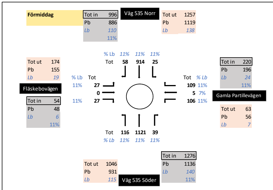
Figur 7 - Dimensionerande trafikflöden i korsningen väg 535-Fläskebovägen-Gamla Partillevägen för förmiddagens maxtimme år 2040, Inklusiv alstring från Link40 med verksamhetstyp "Innovation/omlastning".
