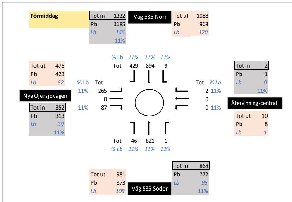
Figur 3 - Dimensionerande trafikflöden i Nya Öjersjörondellen för förmiddagens maxtimme år 2040. Inklusive alstring från Link40 med verksamhetstyp "Innovation/omlastning".
