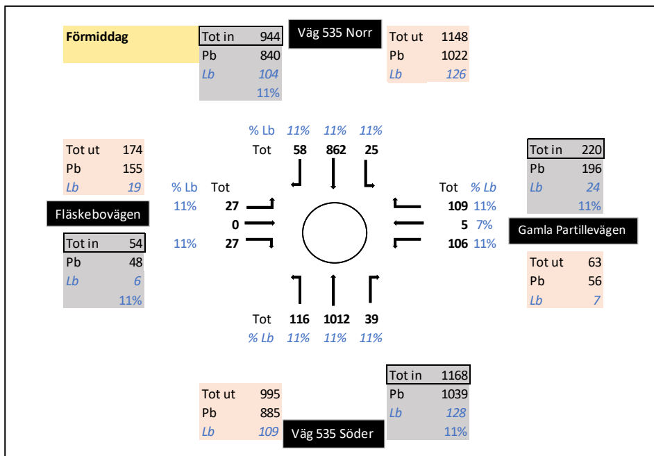
Figur 5 - Dimensionerande trafikflöden i korsningen väg 535-Fläskebovägen-Gamla Partillevägen för förmiddagens maxtimme år 2040, Inklusive alstring från Link40 med verksamhetstyp "Traditionell logistik".
