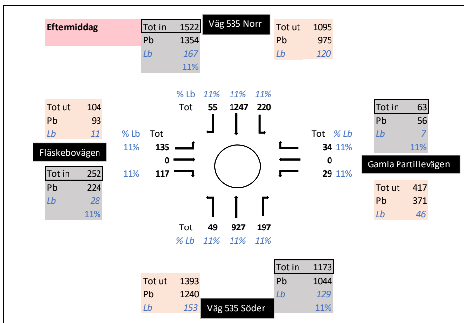
Figur 6 - Dimensionerande trafikflöden i korsningen väg 535-Fläskebovägen-Gamla Partillevägen för eftermiddagens maxtimme år 2040. Inklusive alstring från Link40 med verksamhetstyp "Traditionell logistik".
